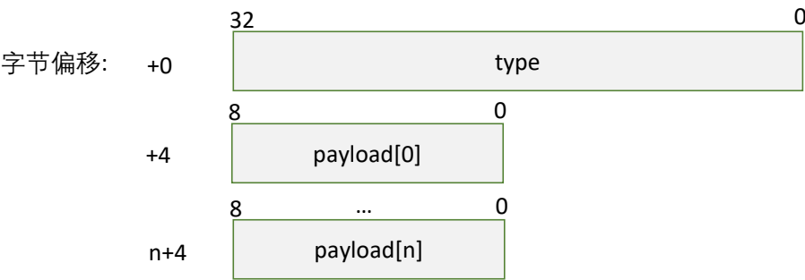
图表 4-26 设备配置信息获取命令请求对应的数据应答报文
