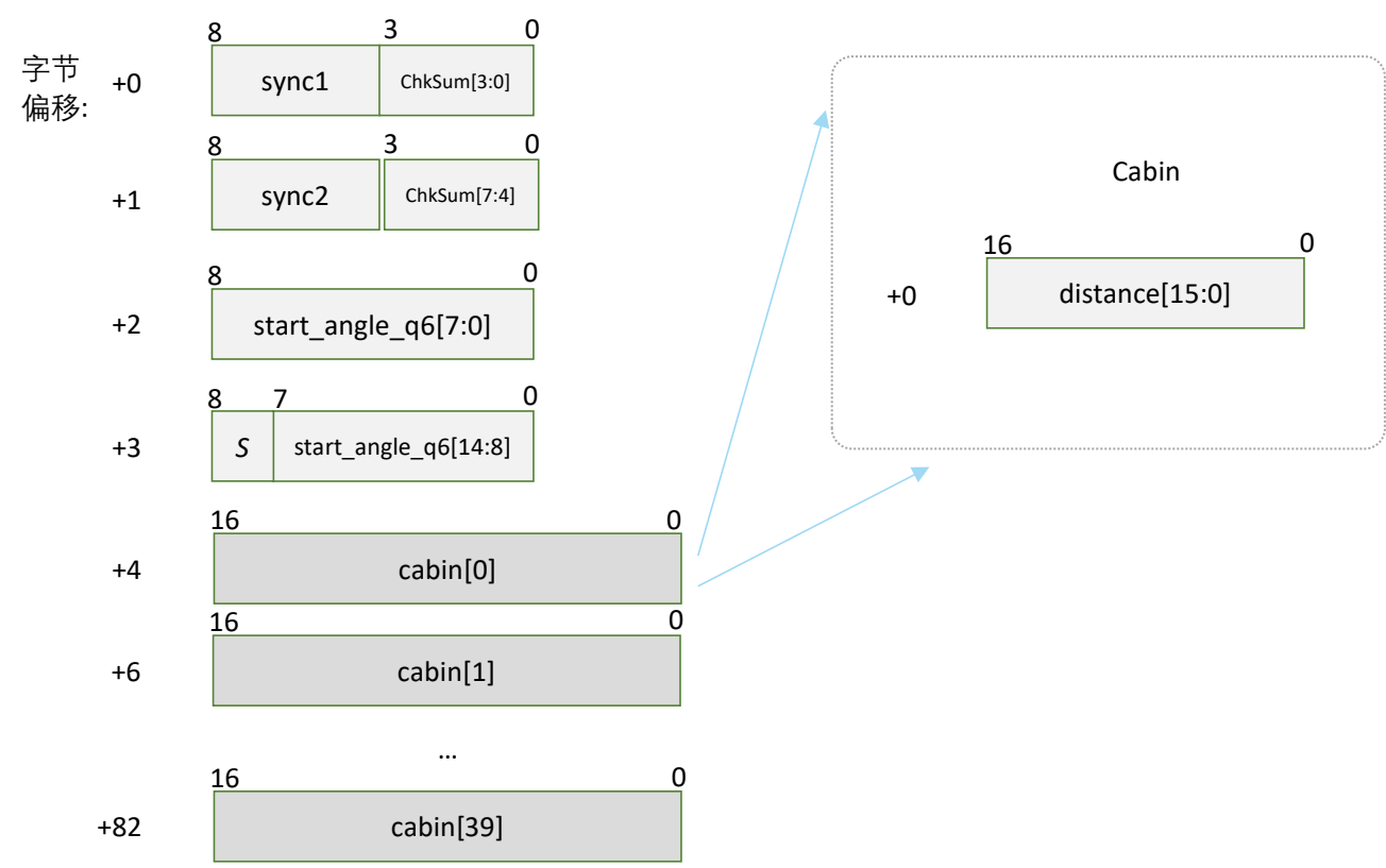
图表 4-12 高速扫描测距输出的数据应答报文格式
