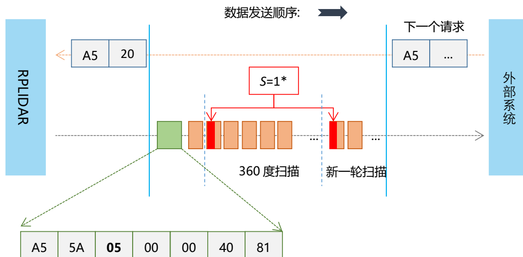
图表 4-9 外部系统发送扫描采样请求后的通讯情况
