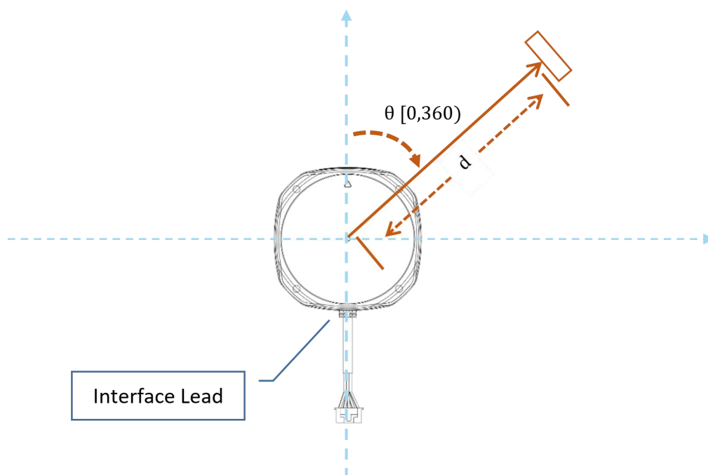
图表 4-7 RPLIDAR S2 测距时夹角与距离值几何定义
