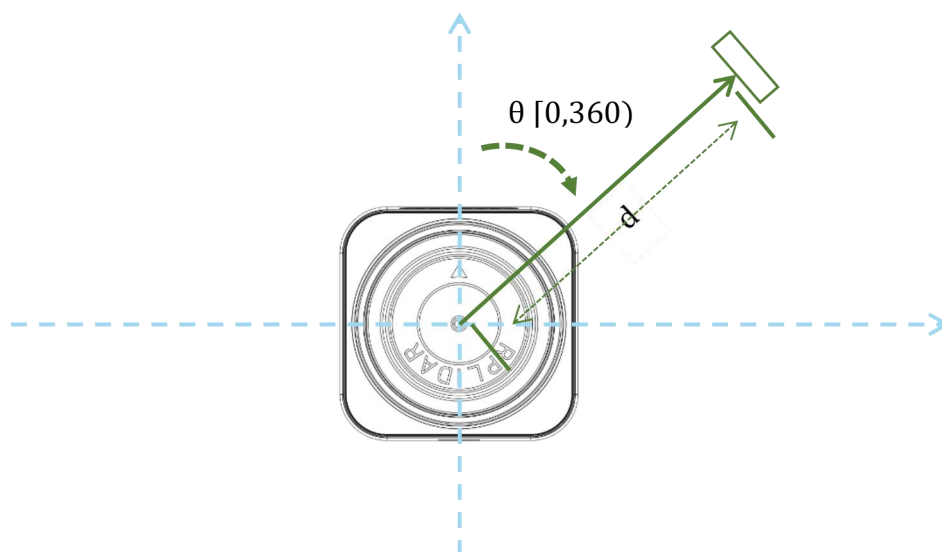
图表 4-6 RPLIDAR S1 测距时夹角与距离值几何定义
