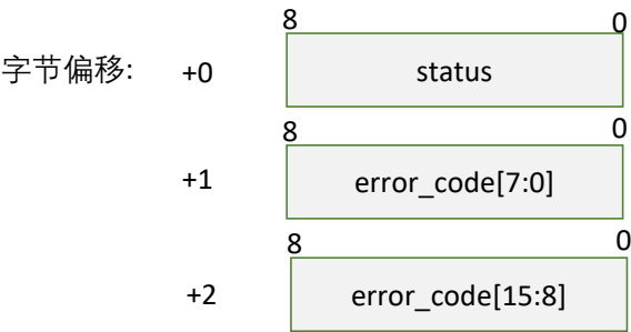
图表 4-20 设备健康状态请求对应的数据应答报文
