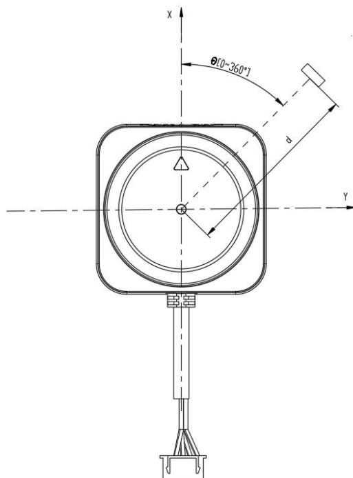
图表 4-8 RPLIDAR S3 测距时夹角与距离值几何定义
