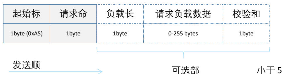
图表 2-4 RPLIDAR 请求报文发送格式
