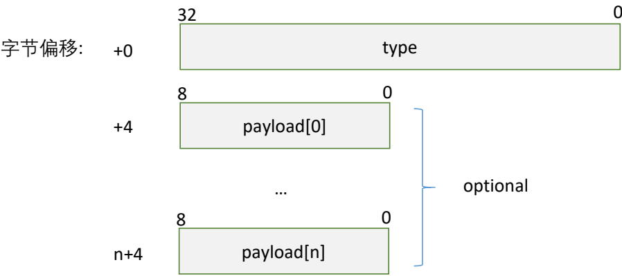
图表 4-24 设备配置信息获取命令请求对应的数据请求报文
