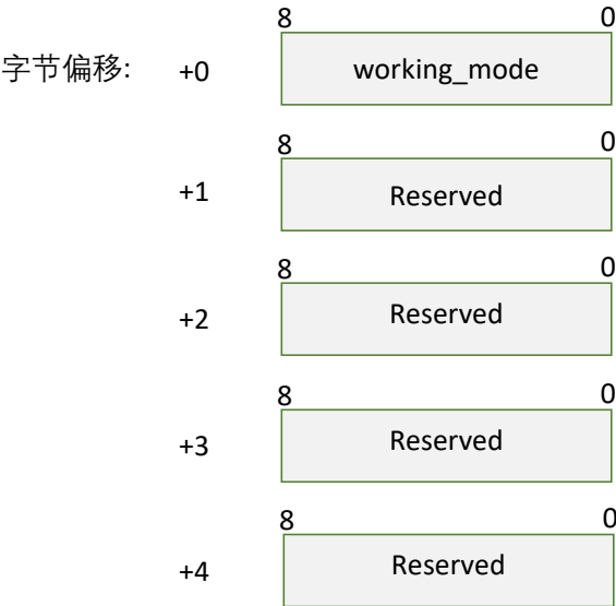
图表 4-10 高速采样模式请求报文的数据格式
