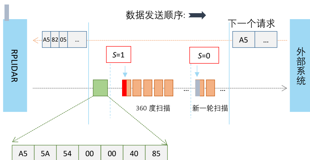
图表 4-15 外部系统在发送高速采样请求后的通讯情况
