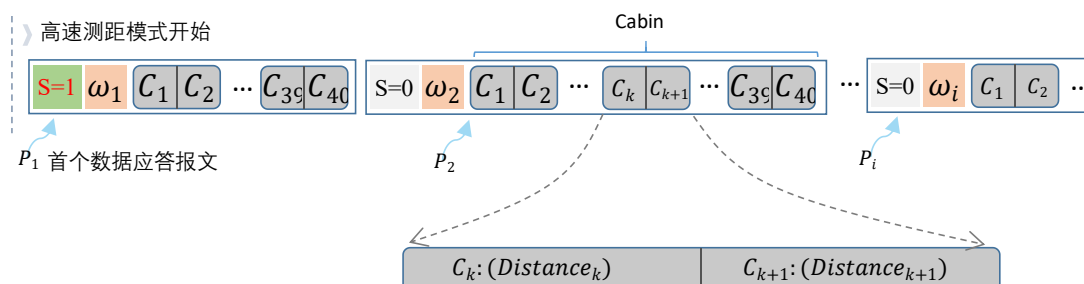
图表 4-16 高速测距模式（密实版本）中发送出的应答报文抽象表示
