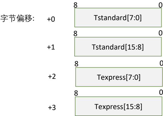
图表 4-22 激光测距用时获取请求对应的数据应答报文
