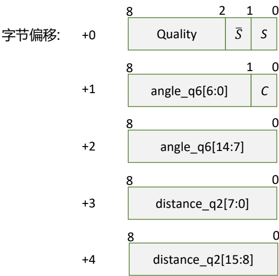
图表 4-4 开始扫描采样 (SCAN) 命令回应数据格式
