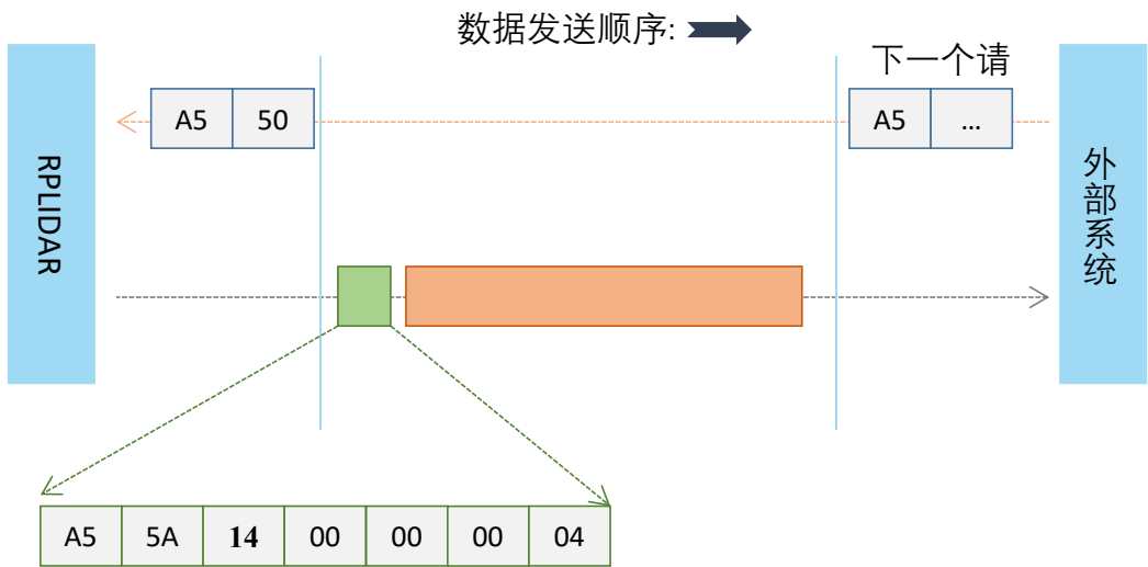
图表 4-19 GET_INFO 请求的通讯时序
