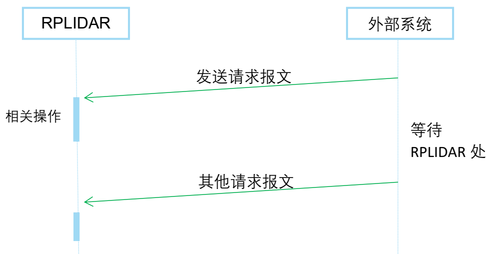
图表 2-3 RPLIDAR 单次请求-无应答模式
