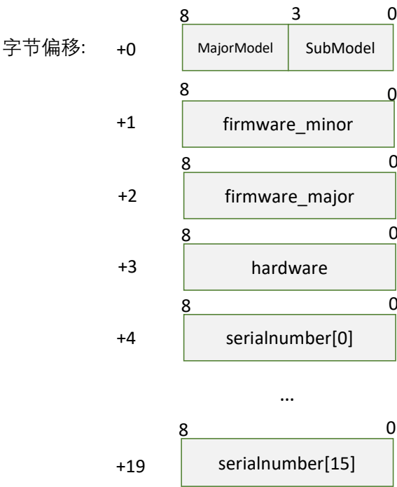
图表 4-17 设备信息获取对应的数据应答报文
