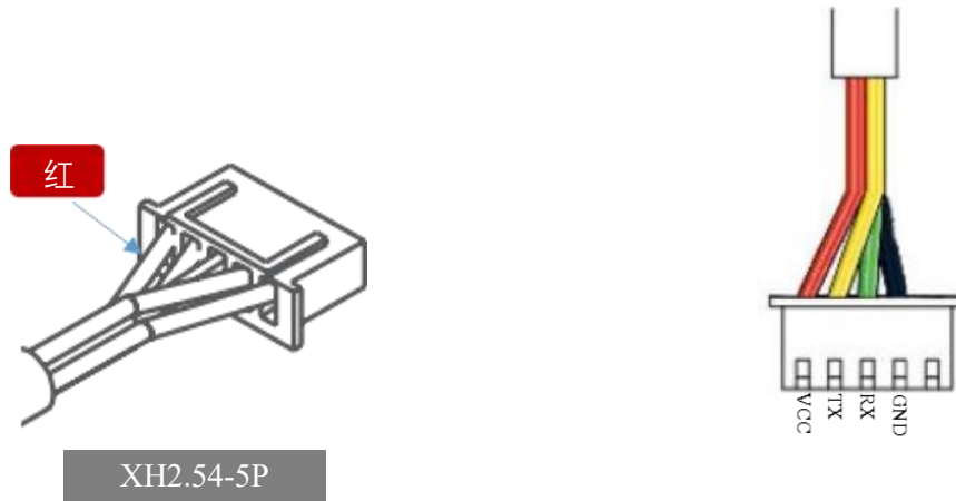
图表 3-1 RPLIDAR S3模块引脚示意图
