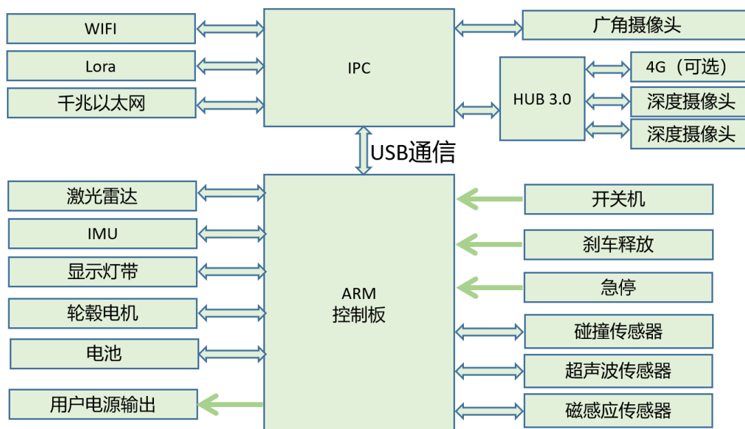
图 3-1 硬件系统框图
